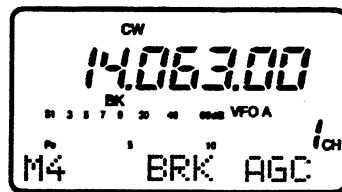
Esempio di selezione del CW con Semi Break-in
